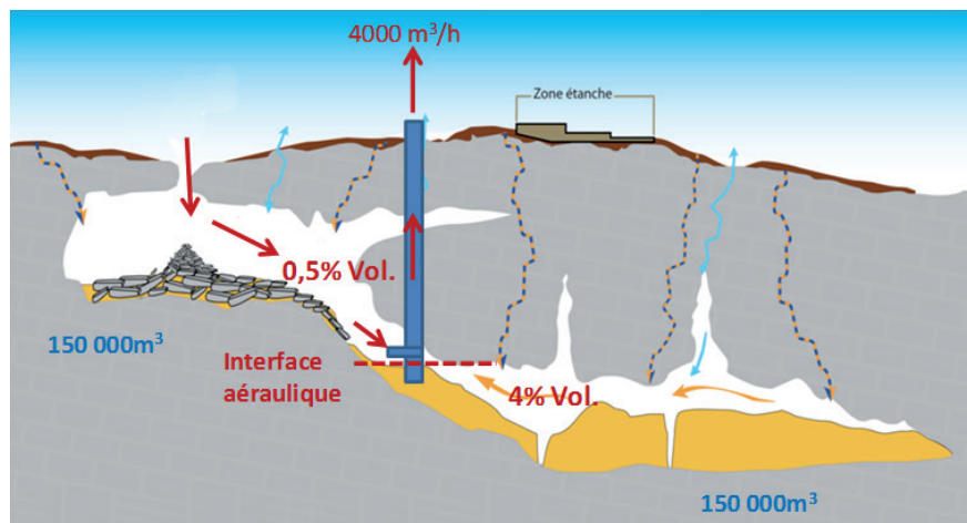
Stimulation de la ventilation dans les galeries supérieures
